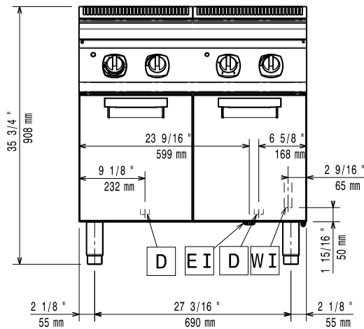
Zij aanzicht
